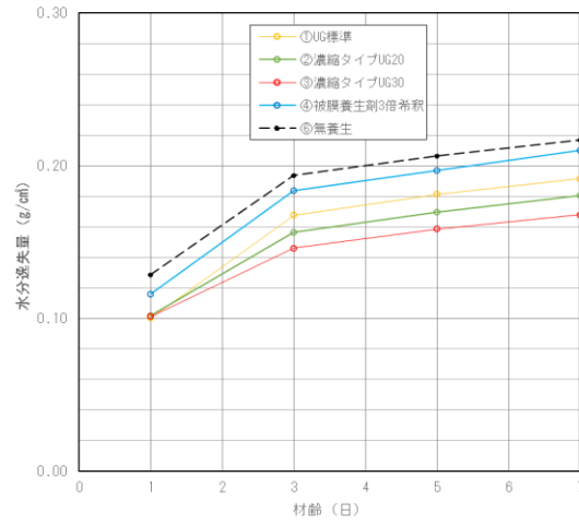
図 養生剤の種類を変えた場合の水分逸失量(g/cm²)試験結果
