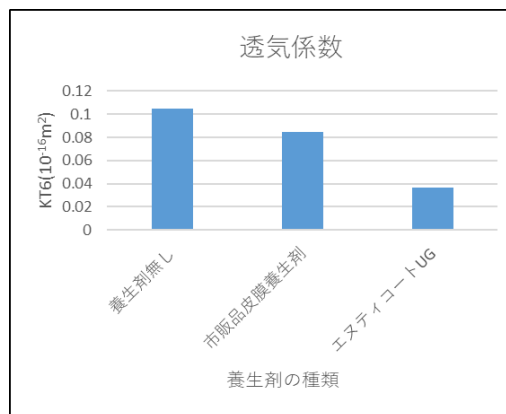
図-2 透気性試験(トレント法によるスイス標準規格 SIA262:2003)
